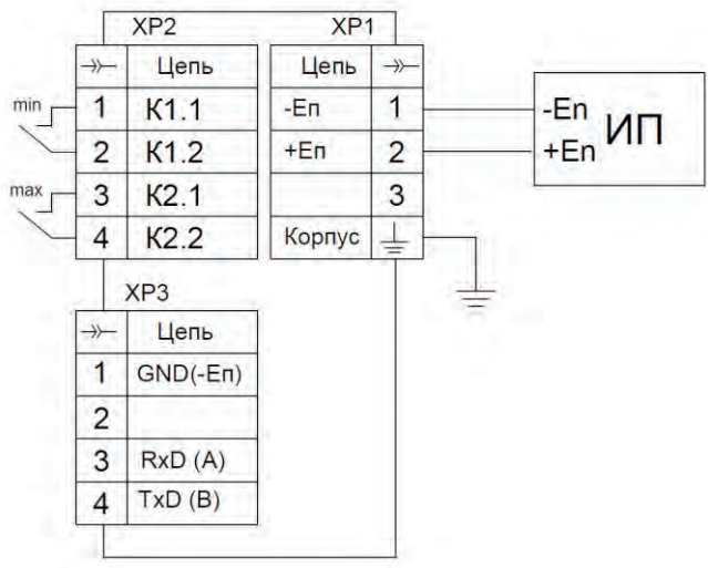
Рисунок В.5 – Прибор ДМ5002М-В
