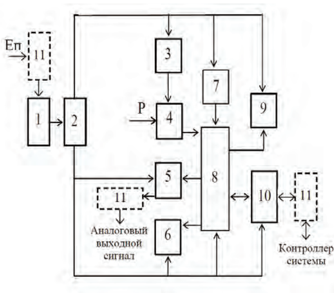
Рисунок 1 – Структурная схема прибора
