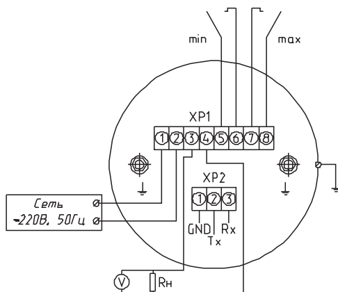
Рисунок В.12 – Прибор ДМС002М-Г 220 В
